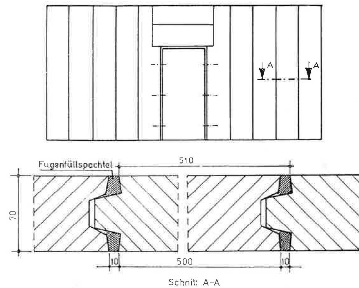
Raumhohe Schaumgips-Streifenplatte
