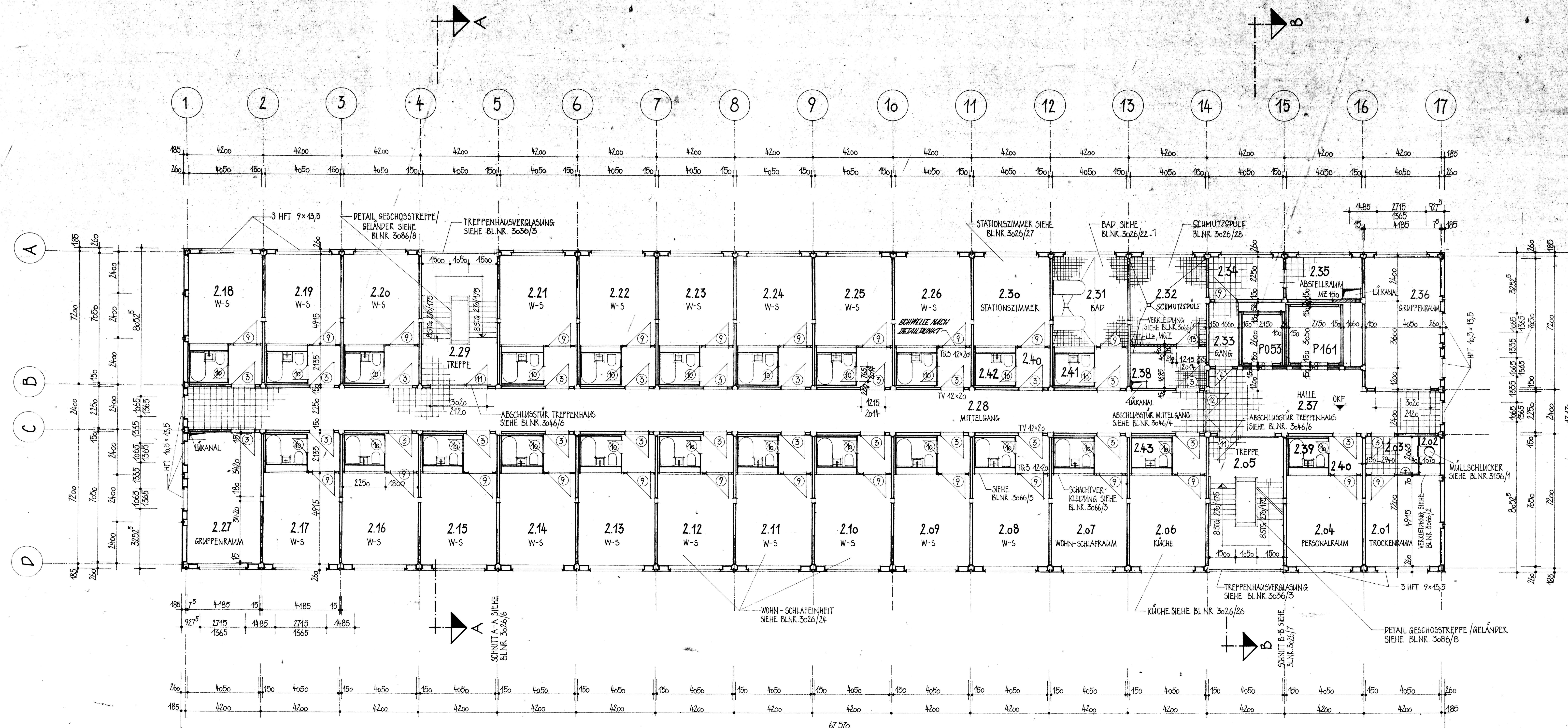
GRUNDRISS 1.u.2. OBERGESCHOSS
