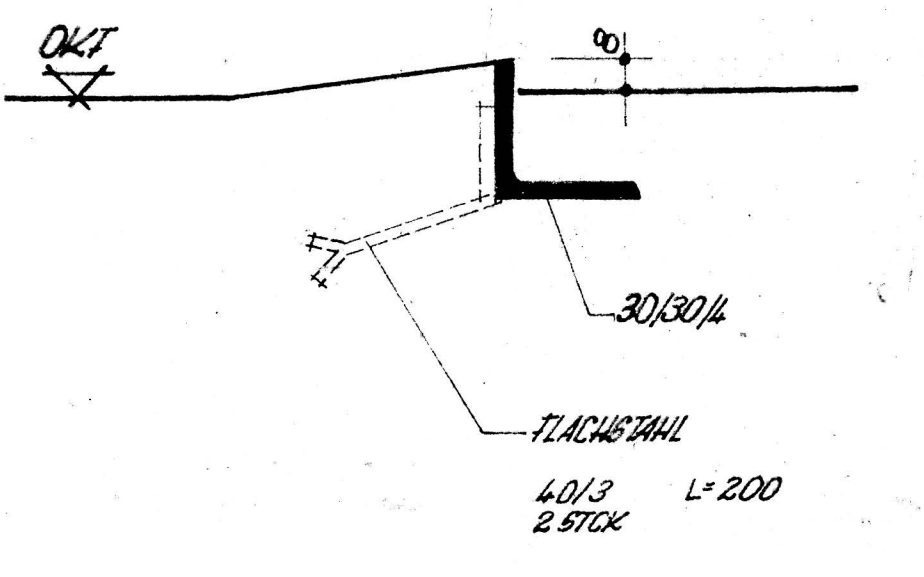
DETAILPUNKT SCHWELLE ZWISCHEN STICHTUR UND WOHNSCHLAFRAUM
