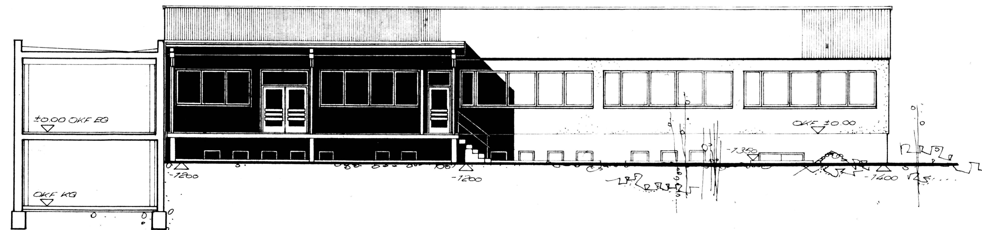
Nord - Ansicht
