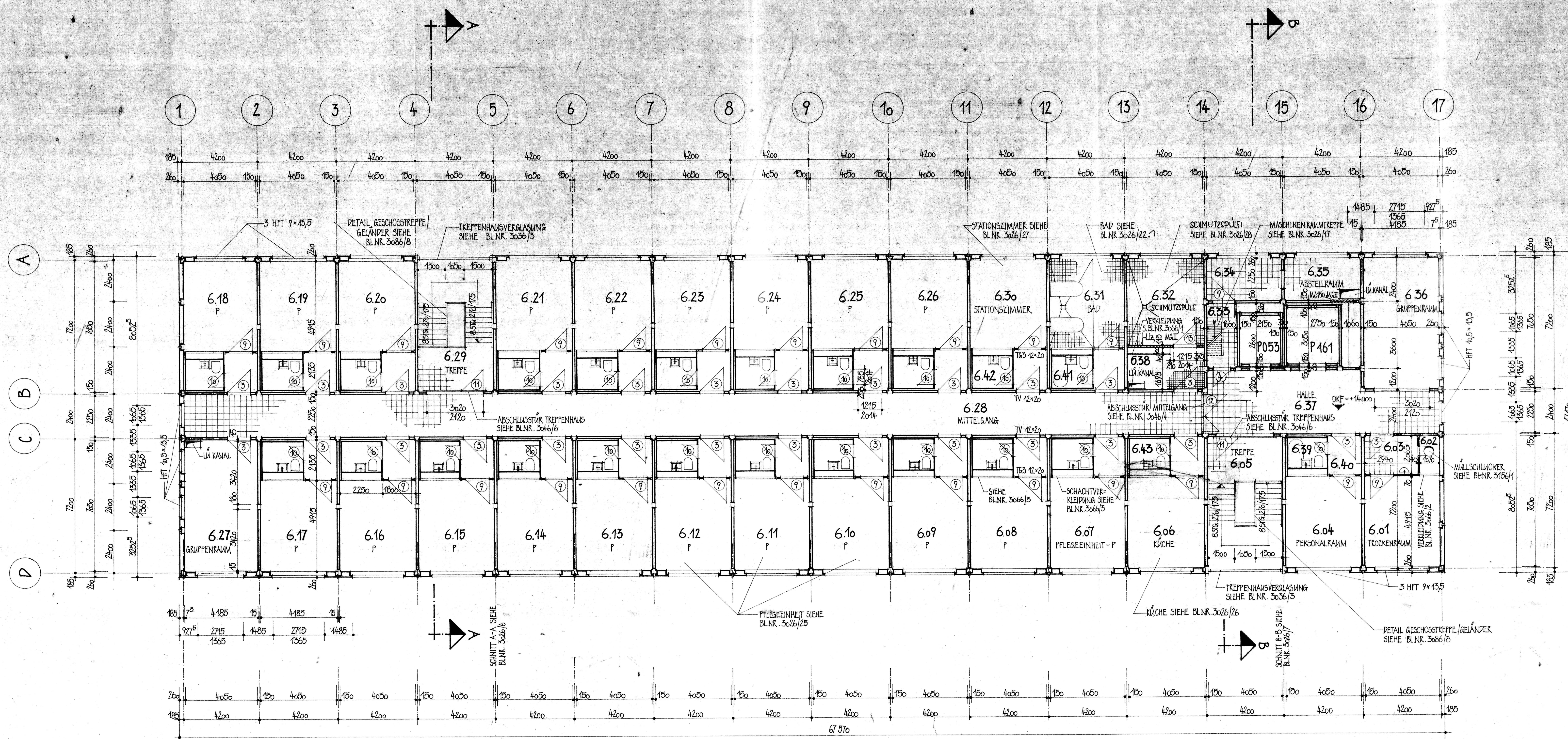
5. OBERGESCHOSS-GRUNDRISS
