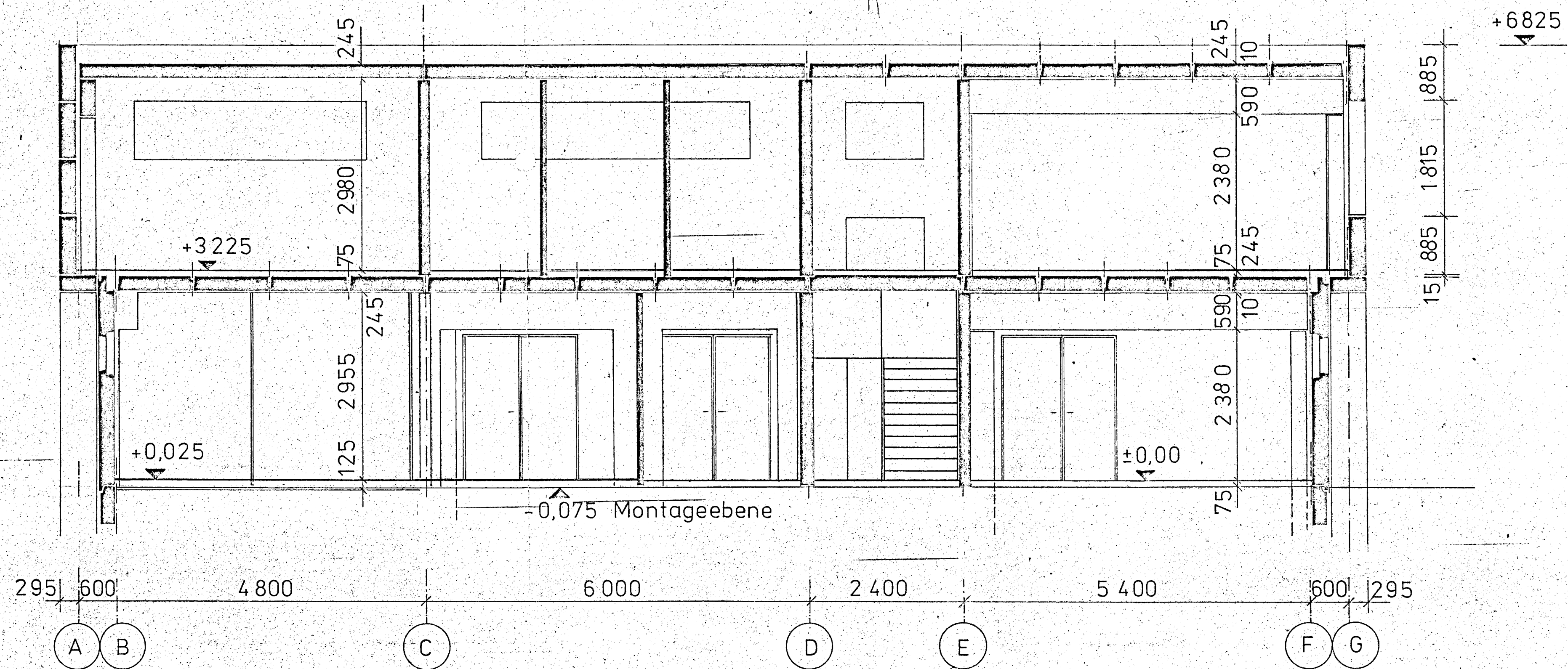
Schnitt C-C
