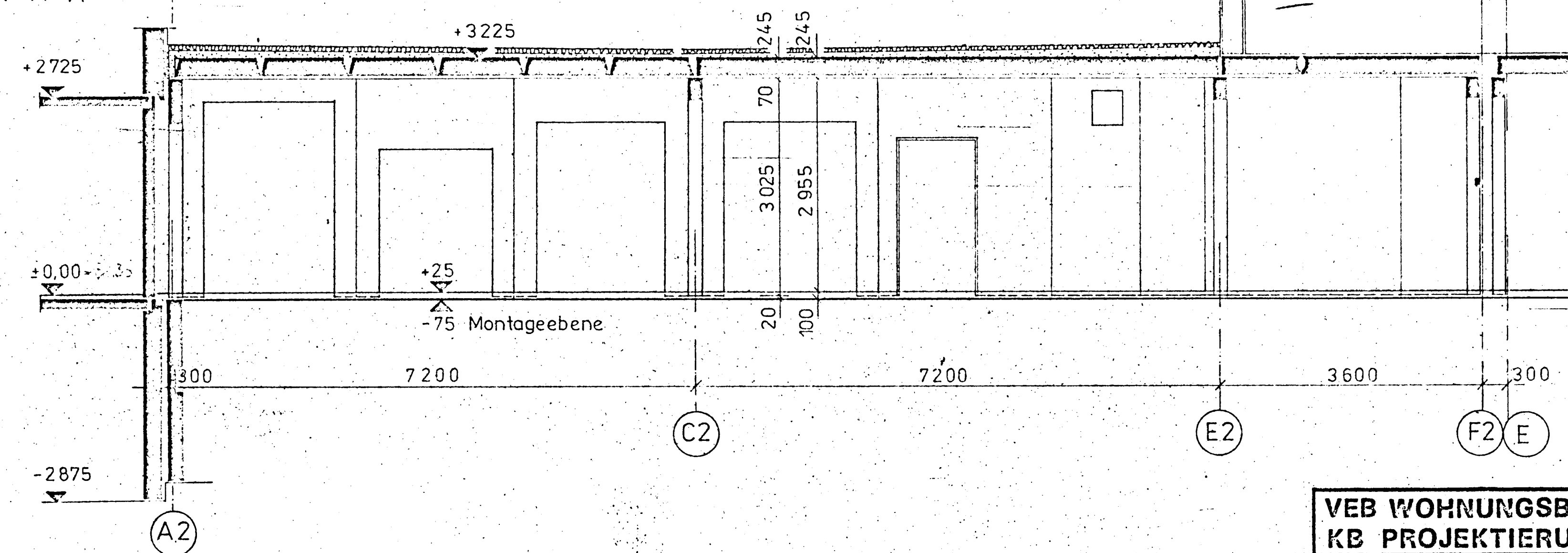
Schnitt B-B
