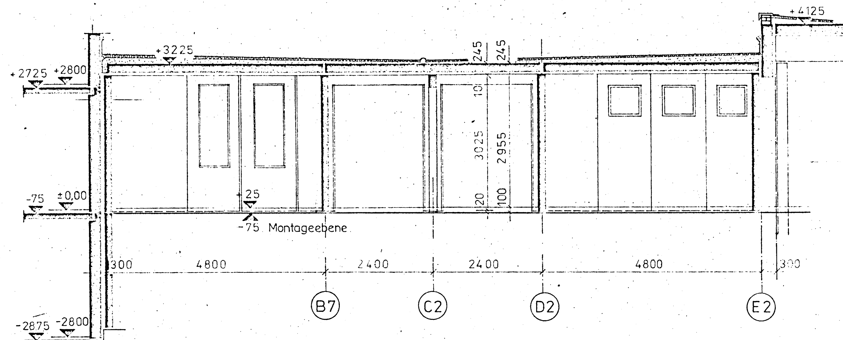
Schnitt A-A
