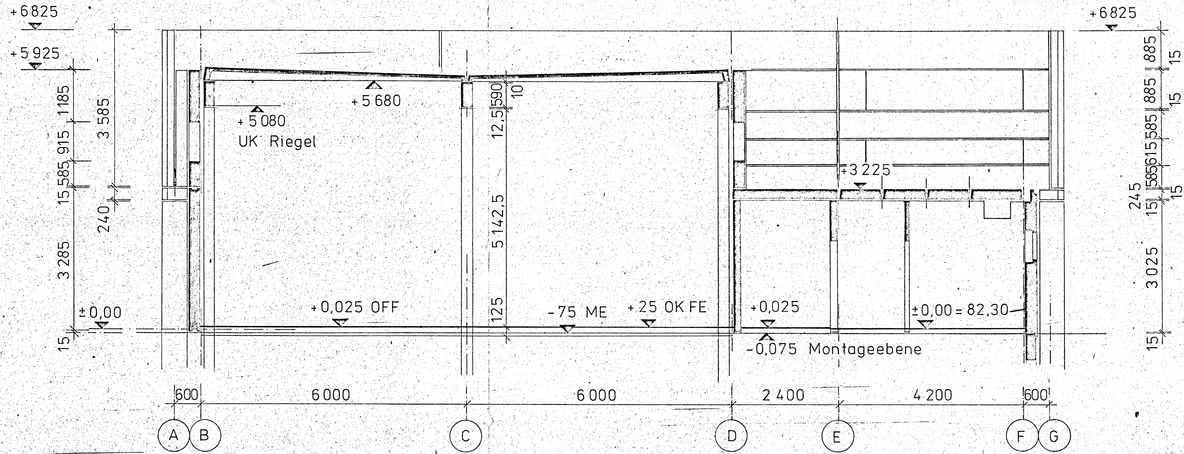
Schnitt D-D
